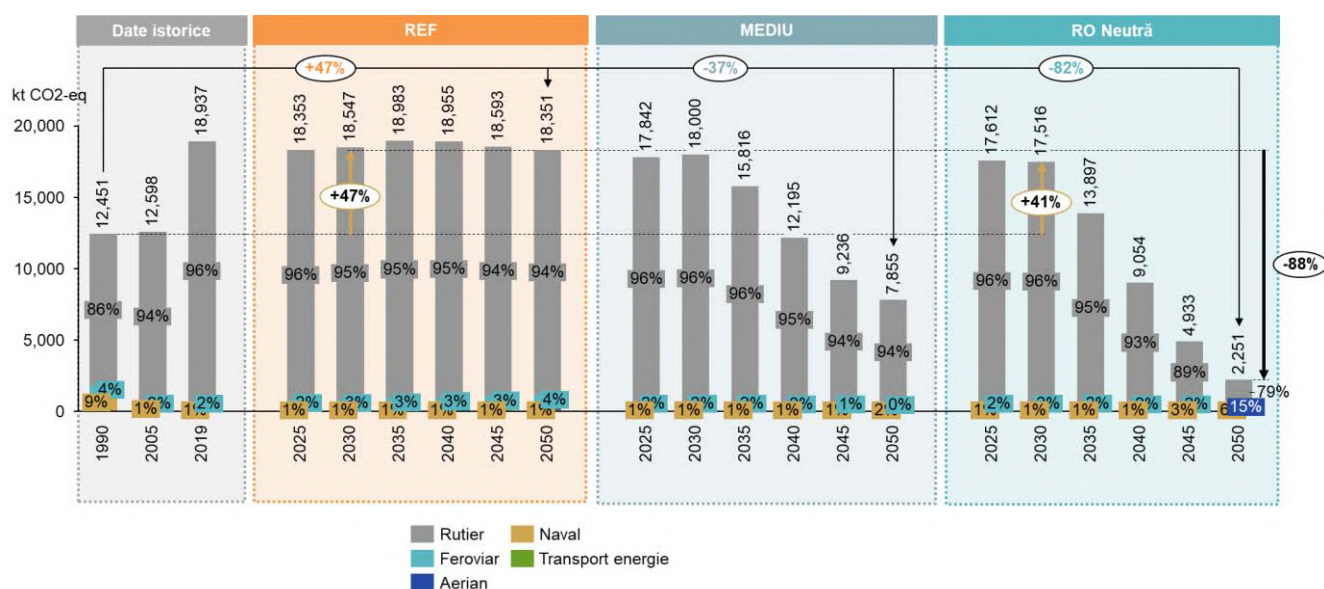
Figura 36. Evoluția emisiilor în domeniul transporturilor per tip de transport conform celor 3 scenarii analizate: REF, Mediu și România Neutră
