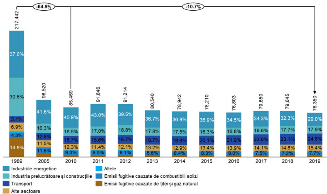
Figura 8. Evoluția emisiilor de GES în sectorul Energie, per domenii (în kt CO 2 -eq), 1989-2019
